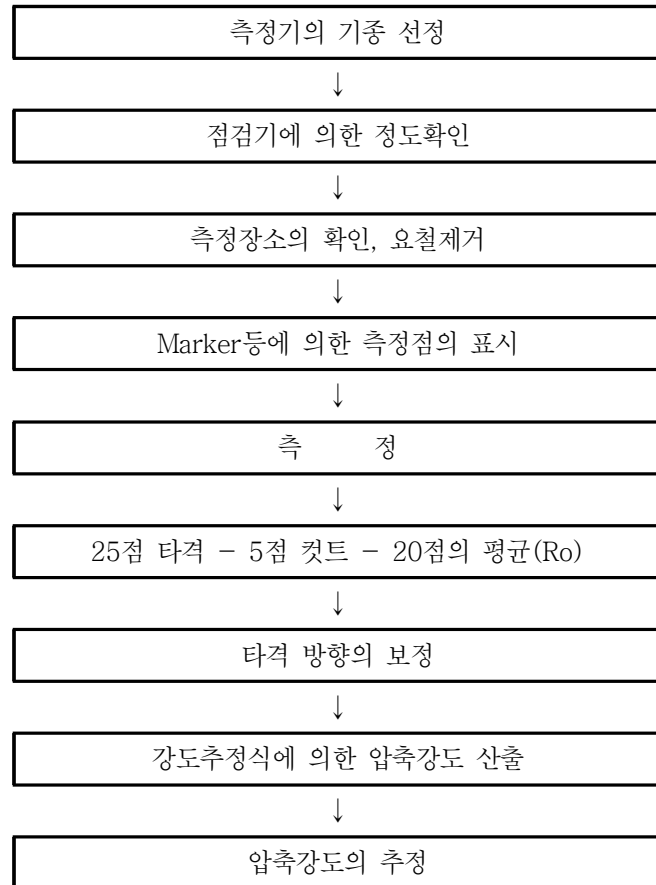
【그림 2.4.1】 반발경도법에 의한 압축강도 추정도
